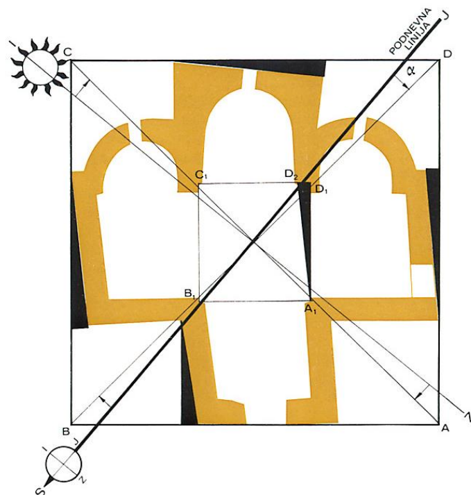
Slika 6. Tlocrt crkve Sv. Križa u Ninu
